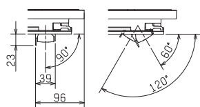
■導風板 (運轉期間 60°至120° 移動範圍)
