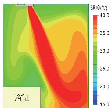
溫度分佈圖
