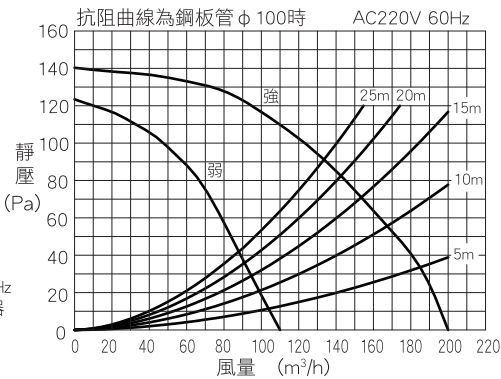
■P-Q特性曲線圖
