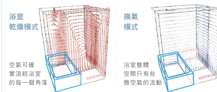
浴室乾燥時的氣流示意圖 (機種：V-141BZ-TWN)
