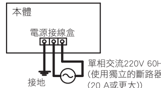
■接線圖
