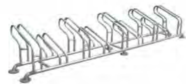
Bicycle Rack •Model : BYE-1111 Size : 3600(W) x 590(D) x 510(H)mm Hot Dip Galvanized •Model : BYEHD-2222 Size : 3600(W) x 590(D) x 510(H)mm
