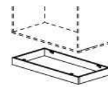
BASE GB 880 795W x 385D x 85H
