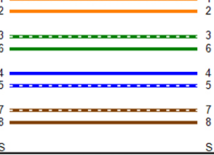
接線圖 (T568B)
