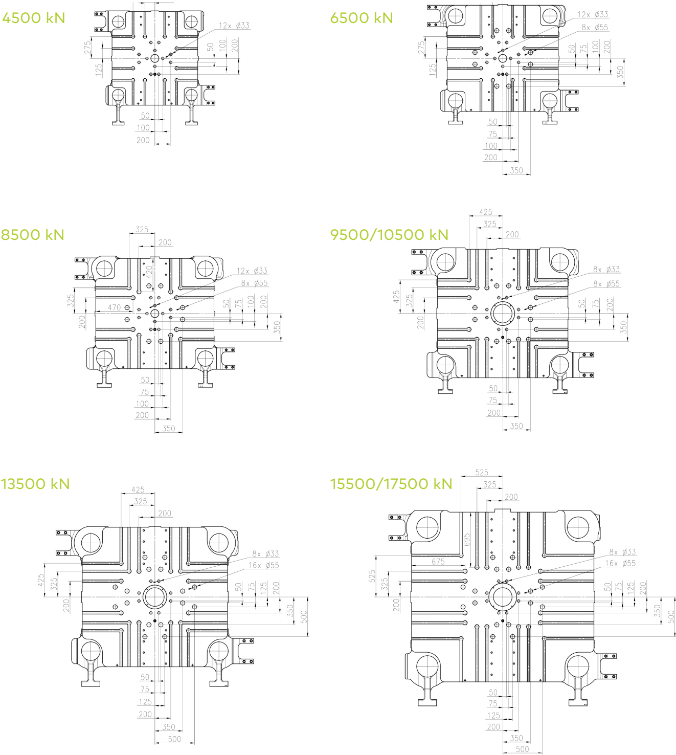
t-win Platen Dimesions 模板尺寸
