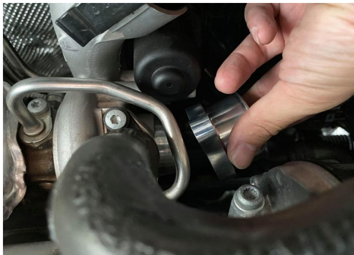
Figure 10: 安裝MST轉接座至渦輪位置(注意螺絲孔位方向)
