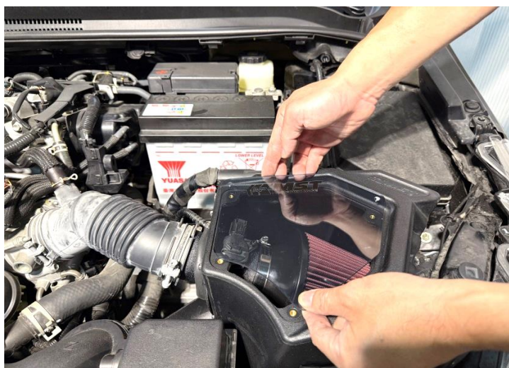
步驟 17: 安裝集氣箱上蓋 使用M4螺絲鎖緊
