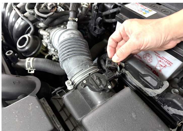
步驟 2: 斷開MAF接頭
