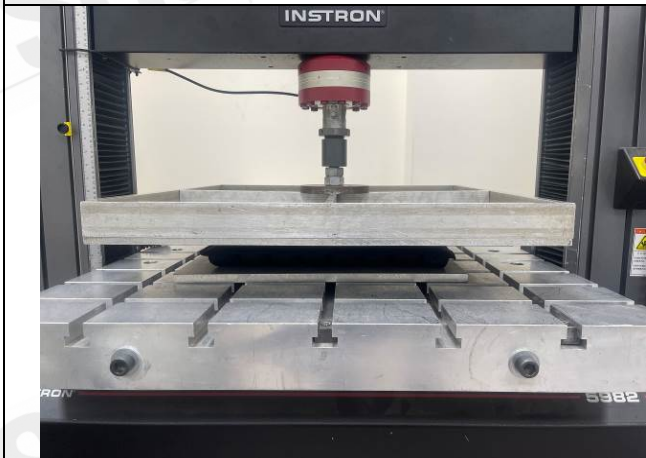
照片 G：測試架設 (樣品#2)
