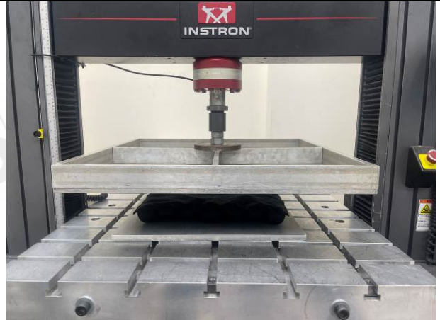
照片 F：測試架設 (樣品#1)
