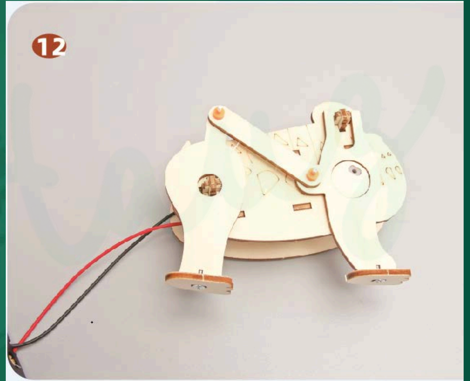
如图安装前部圆孔卡在马达上
