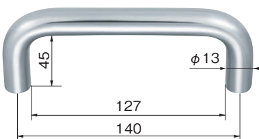
A-1042特注取手SEMI-S8規格φ13仕様 SEMI S8-0218準拠品 (クリーンルーム用手袋着用時)
